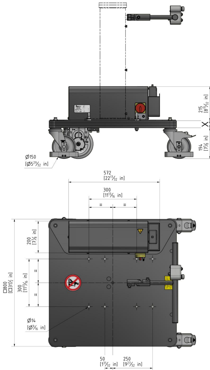
Carrello elettrico - 800x800
