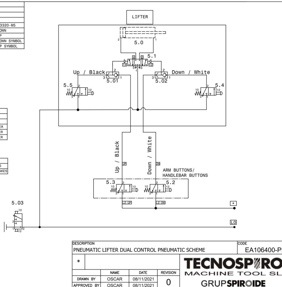
Pneumatischer Heber – Doppelantrieb
