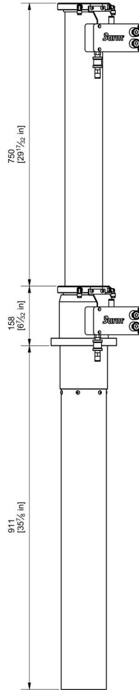
Pneumatischer Heber 750
