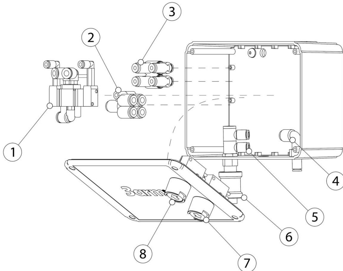
Pneumatischer Heber – Doppelantrieb
