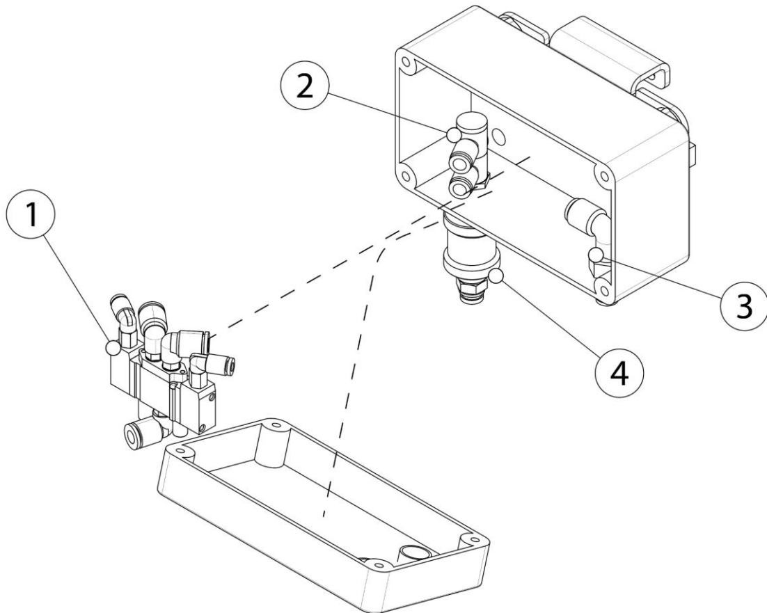
Pneumatischer Heber – ohne Antrieb (externer Antrieb)
