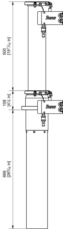
Pneumatischer Heber 500
