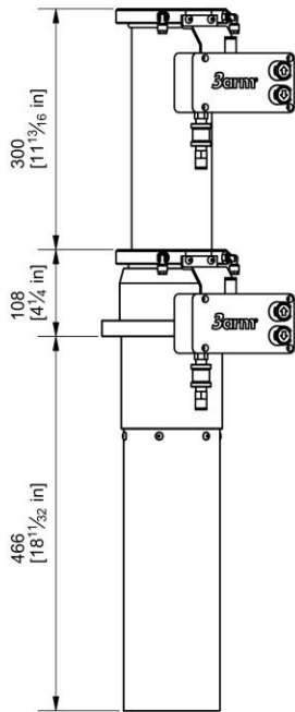
Pneumatischer Heber 300
