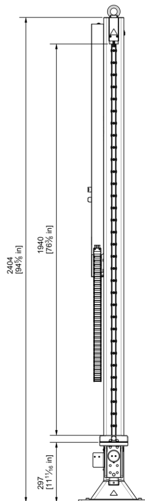
Élévateur 2500 D63
