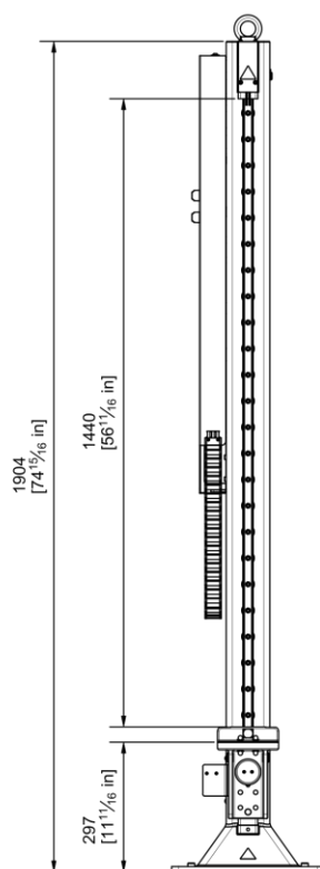
Élévateur 2000 D63
