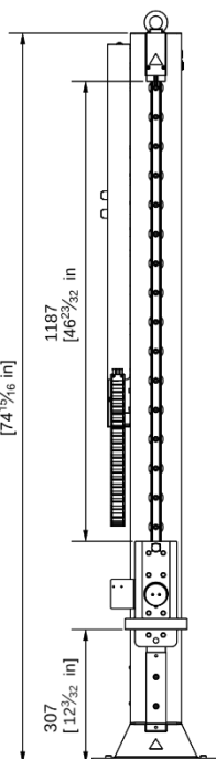
Élévateur 2000 D63 au plafond
