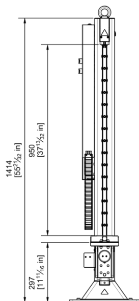
Élévateur 1500 D63
