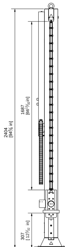
Élévateur 2500 D63 au plafond
