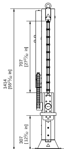
Élévateur 1500 D63 au plafond
